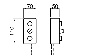
PULSANTIERA DI PIANO (SCALA 1/10)
